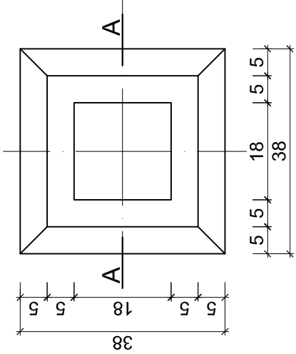
STOPA FUNDAMENTOWA - 14 szt + 1szt pod krzyż prawosławny
