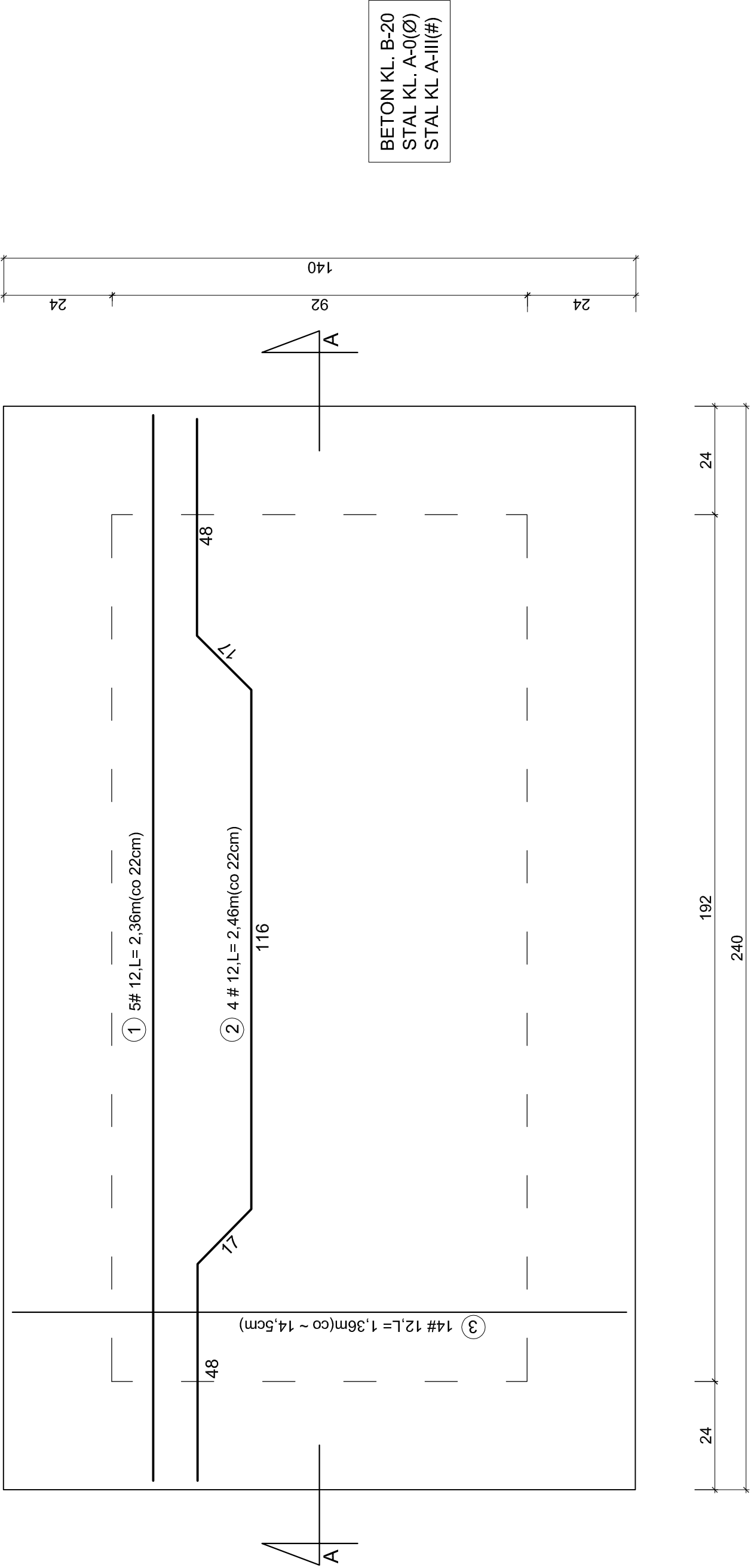
ZESTAWIENIE STALI ZBROJENIOWEJ
