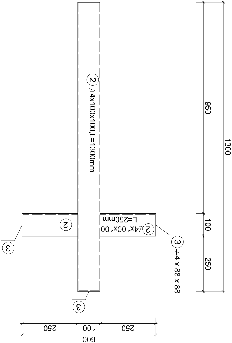
KRZYŻ KATOLICKI POJEDYNCZY - 117 szt
