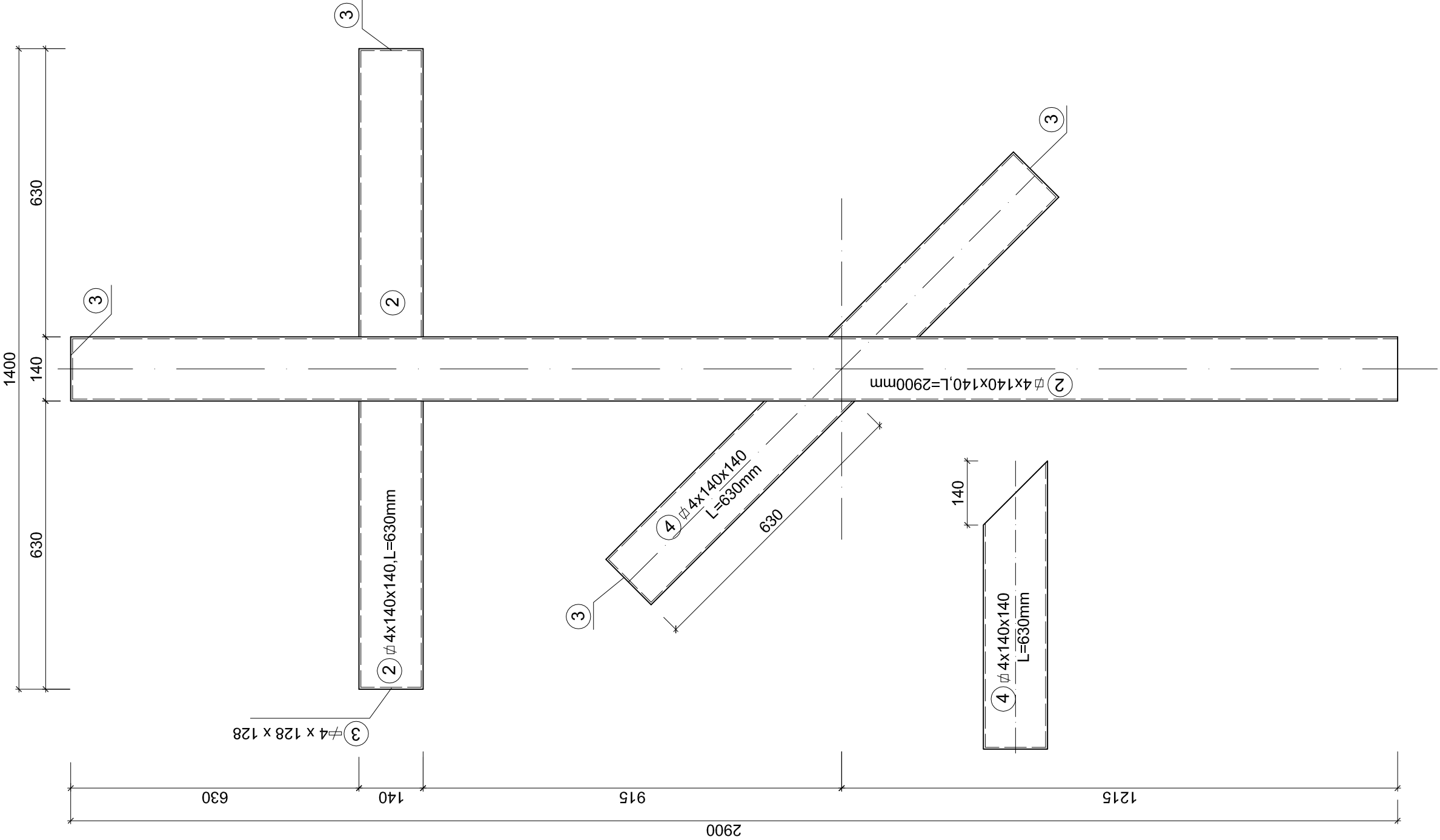
STOPA FUNDAMENTOWA - 5 szt +39 szt pod krzyż katolicki
